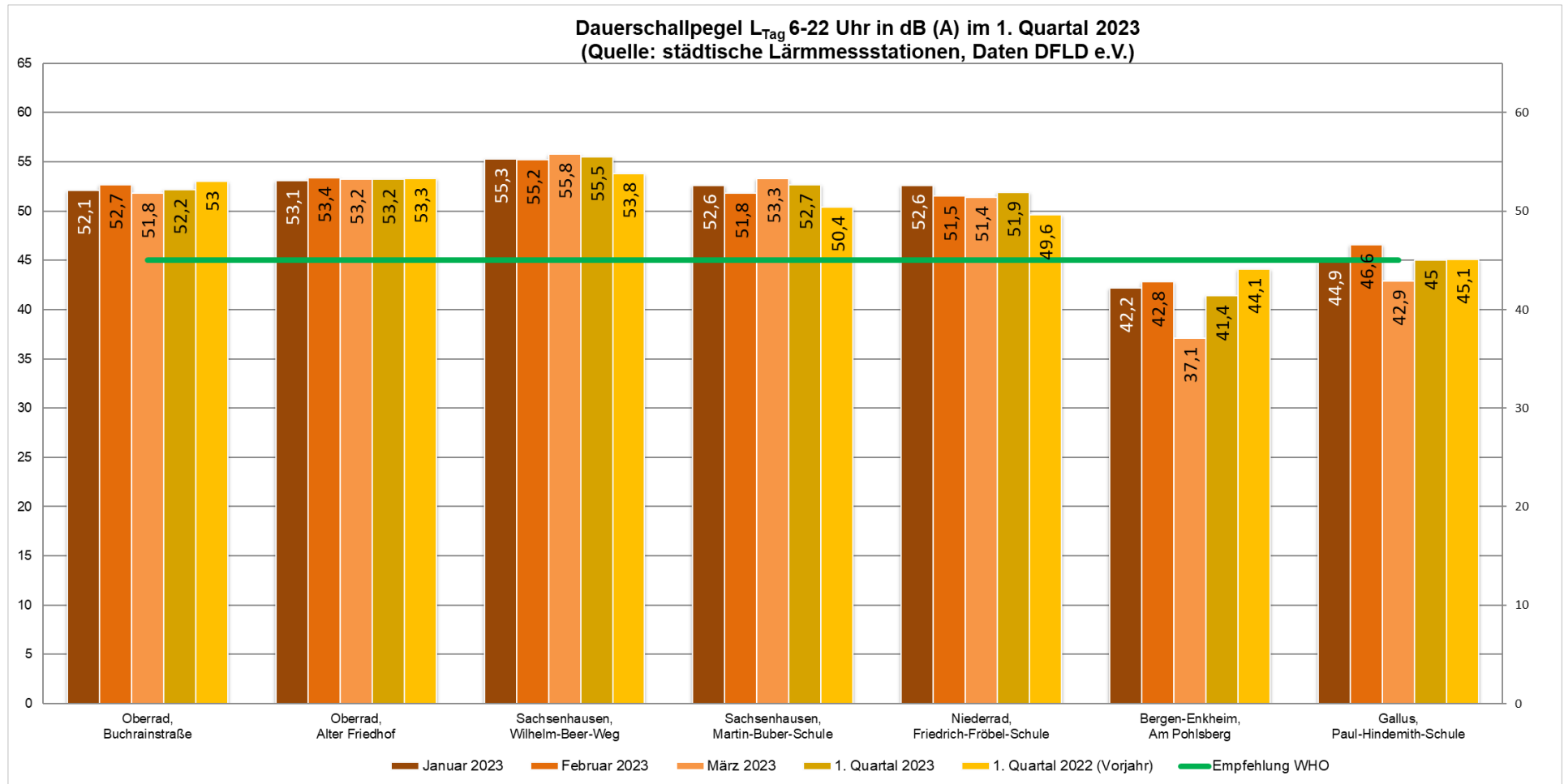
Diagramm 3: Dauerschallpegel L_{\text{Tag}} der städtischen Lärmmessstationen im 1. Quartal 2023 im Vergleich zum 1. Quartal 2022
