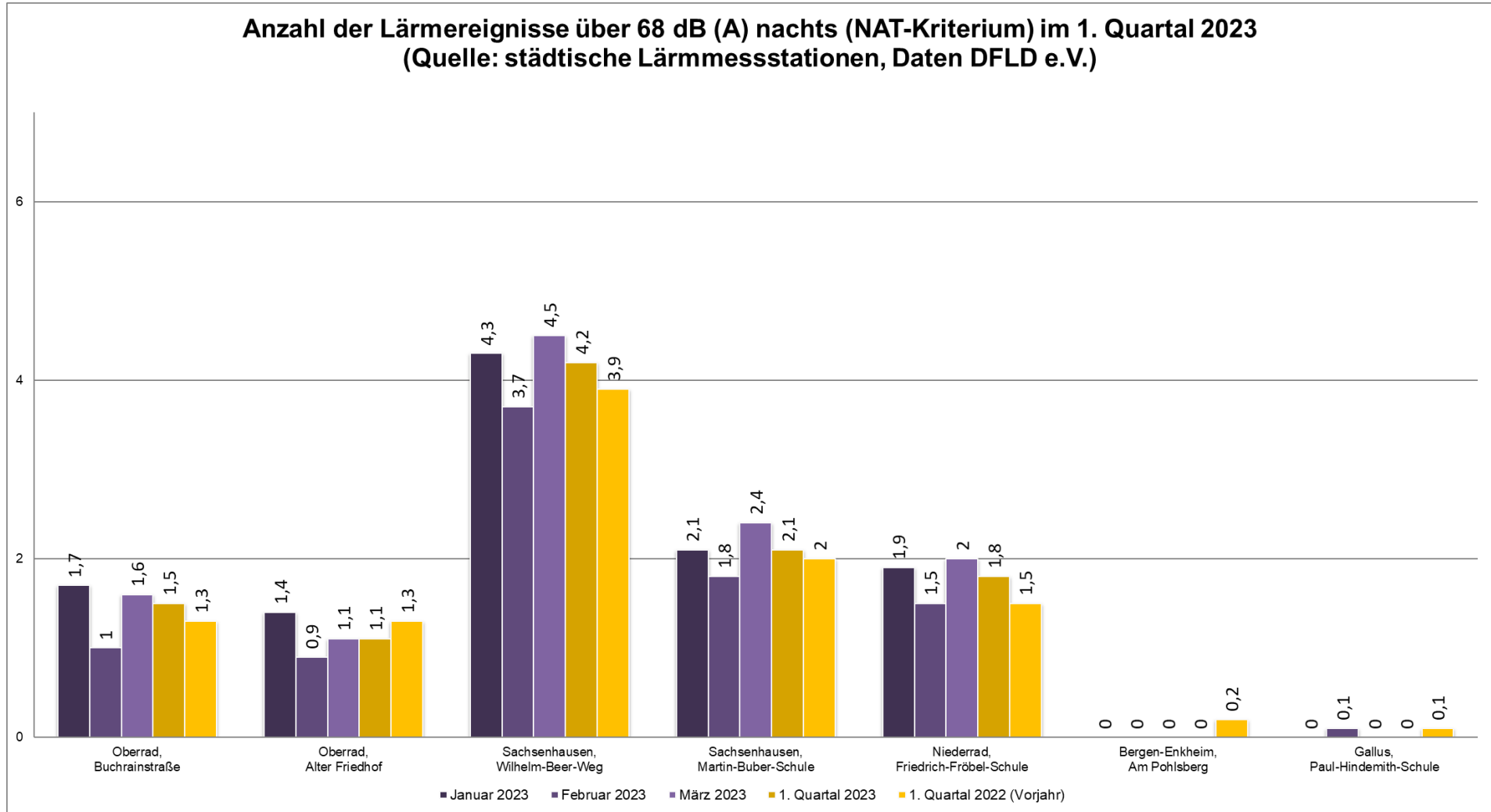
Diagramm 6: durchschnittliche Anzahl der Lärmereignisse über 68 dB (A) nachts (NAT-Kriterium) im 1. Quartal 2023 im Vergleich zum 1. Quartal 2022
