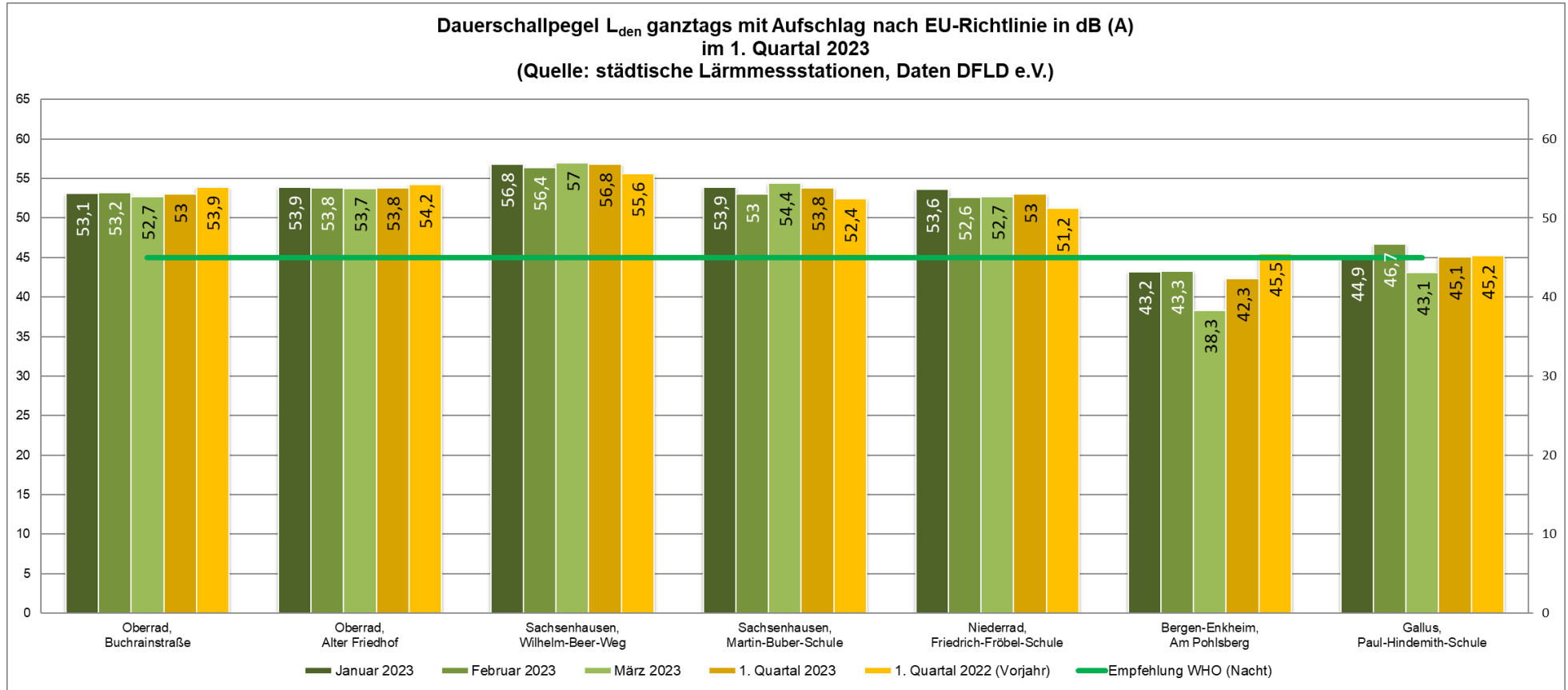
Diagramm 5: Dauerschallpegel L_{den} der städtischen Lärmmessstationen im 1. Quartal 2023 im Vergleich zum 1. Quartal 2022
