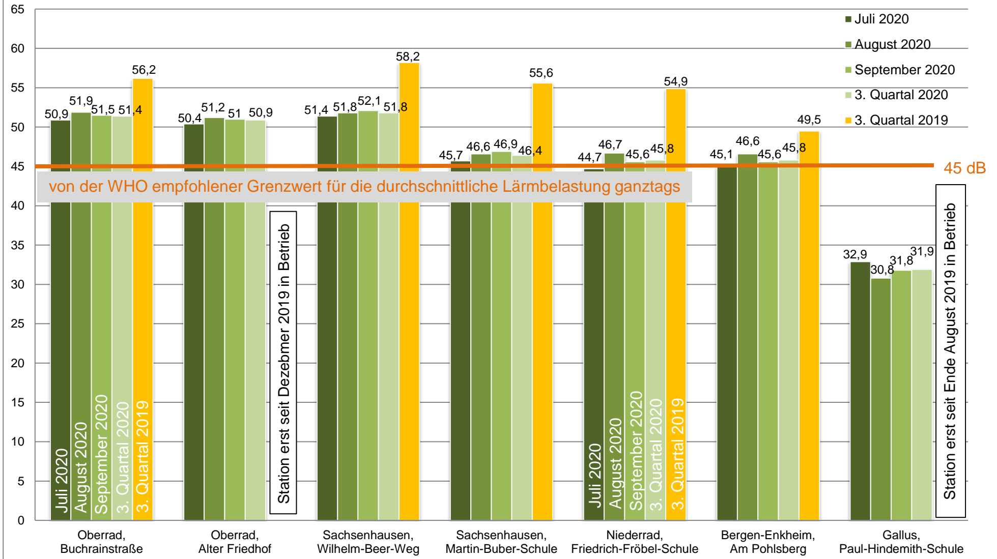
Diagramm 5: Dauerschallpegel L_{den} der städtischen Lärmmessstationen im 3. Quartal 2020 im Vergleich zum Jahr 2019
