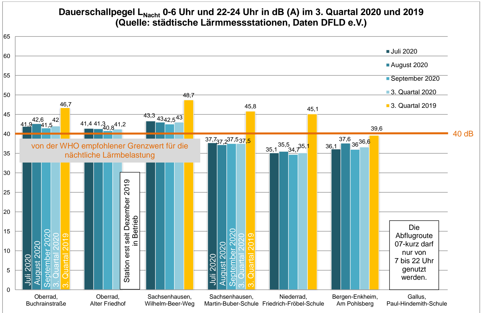
Diagramm 4: Dauerschallpegel L_{\text{Nacht}} der städtischen Lärmmessstationen im 3. Quartal 2020 im Vergleich zum Jahr 2019
