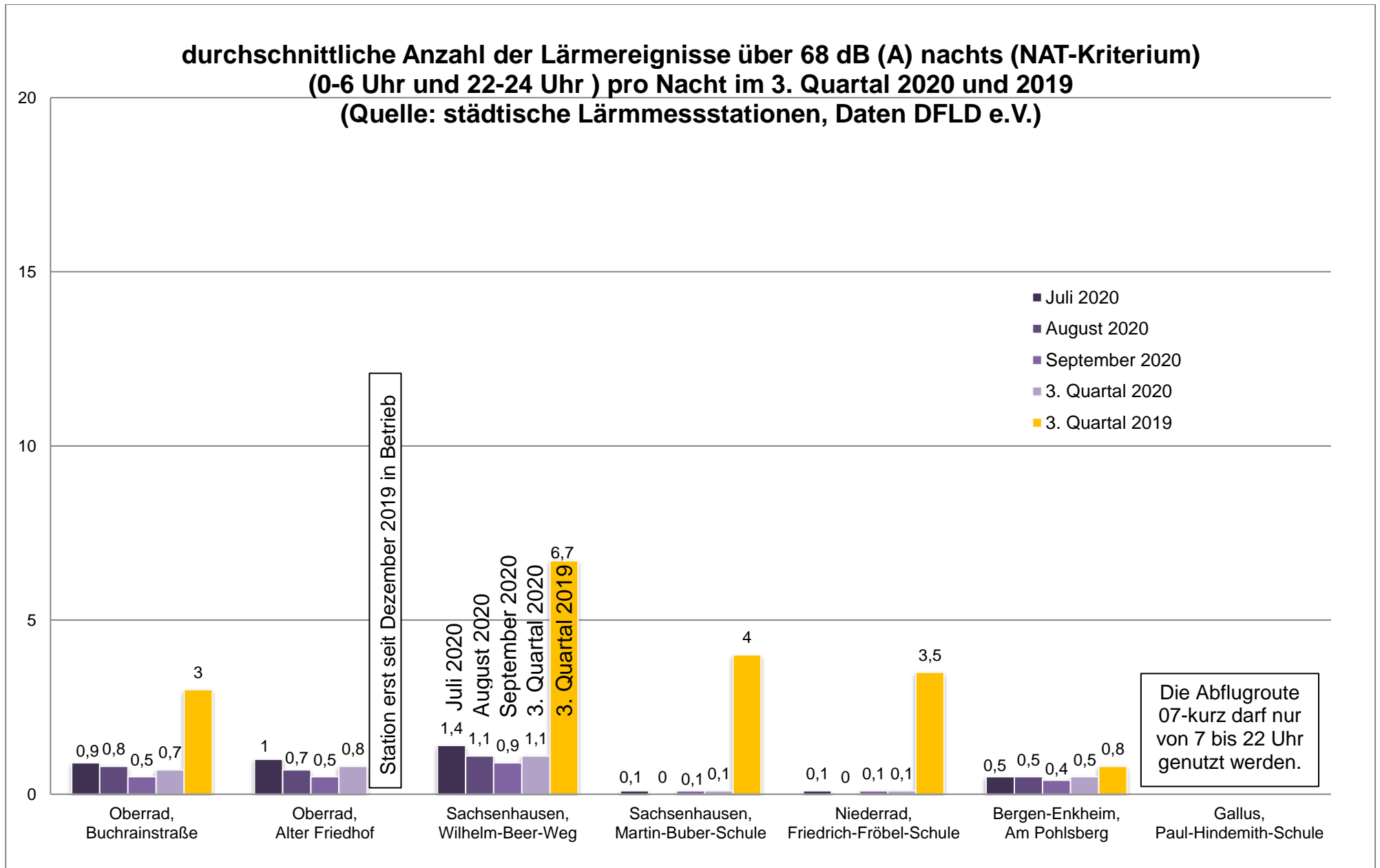
Diagramm 6: durchschnittliche Anzahl der Lärmereignisse über 68 dB (A) nachts (NAT-Kriterium) im 3. Quartal 2020 im Vergleich zum Jahr 2019
