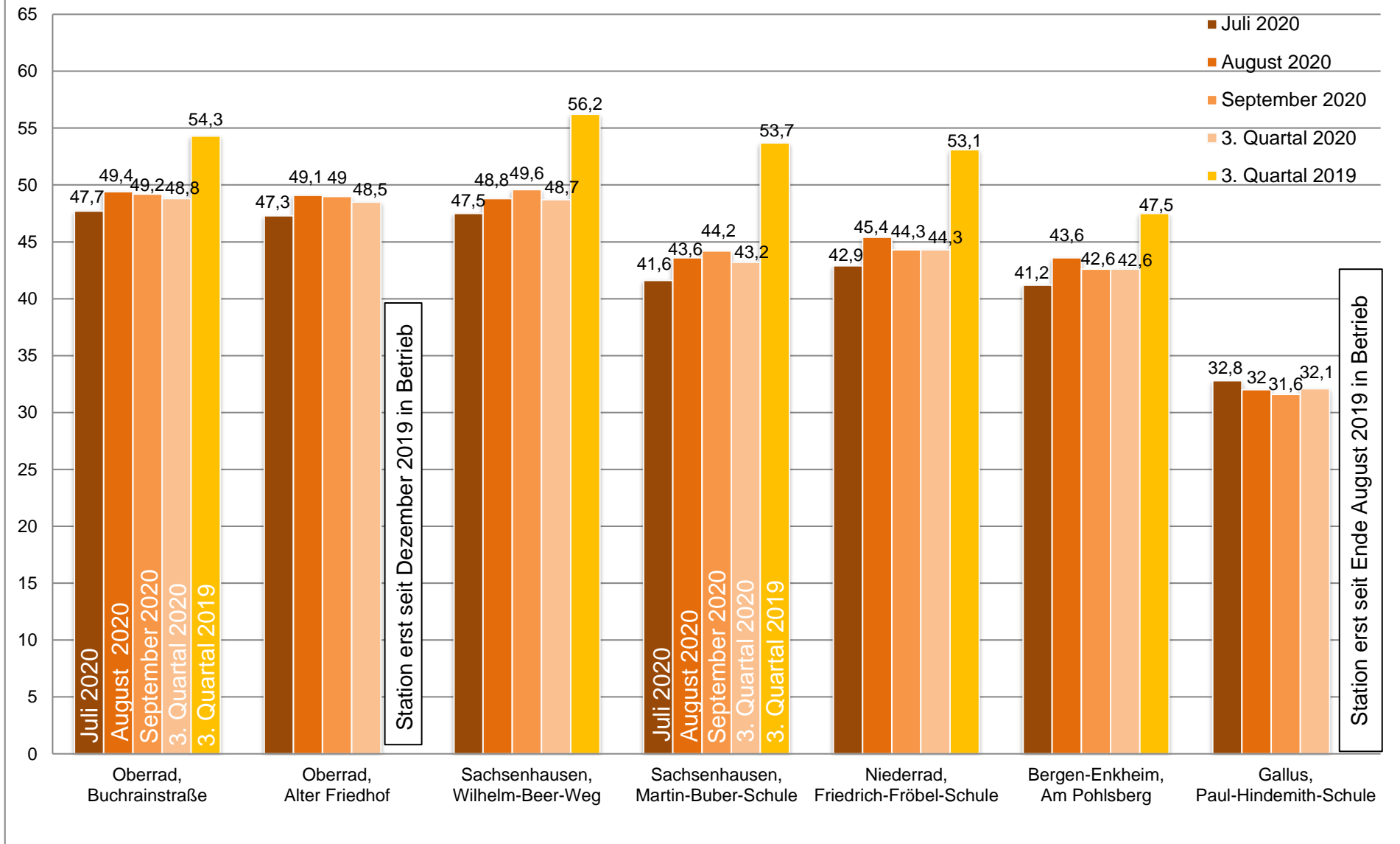
Diagramm 3: Dauerschallpegel L_{\text{Tag}} der städtischen Lärmmessstationen im 3. Quartal 2020 im Vergleich zum Jahr 2019
