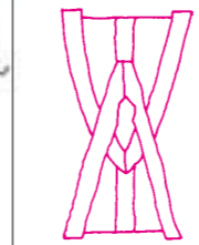
Bundständer in Gestalt verschiedener Verstrebnungsfiguren
