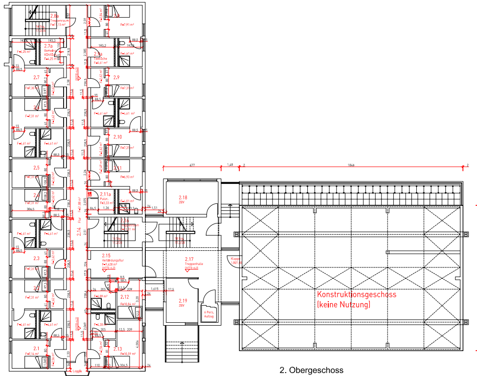
2. Obergeschoss
