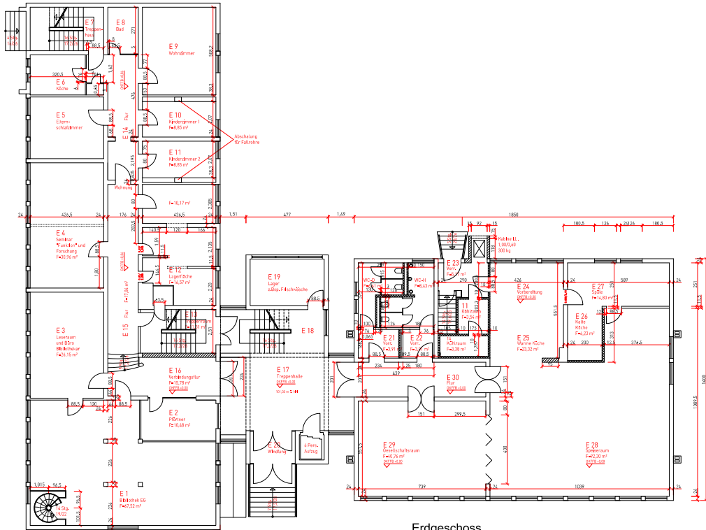
Erdgeschoss
